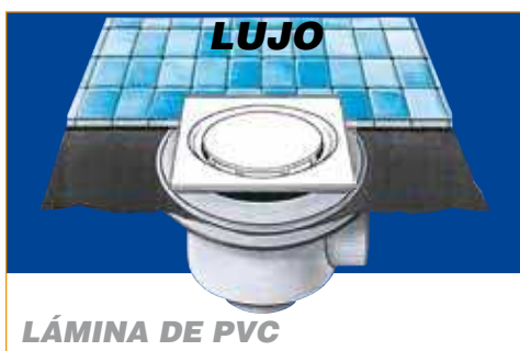
VÁLVULA PLATO DE DUCHA OBRA LUJO "DELUXE" VALVE FOR BUILDING SHOWER BASE
